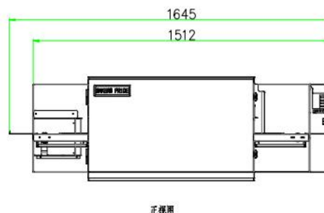
正视图
