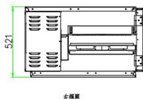
左视图
